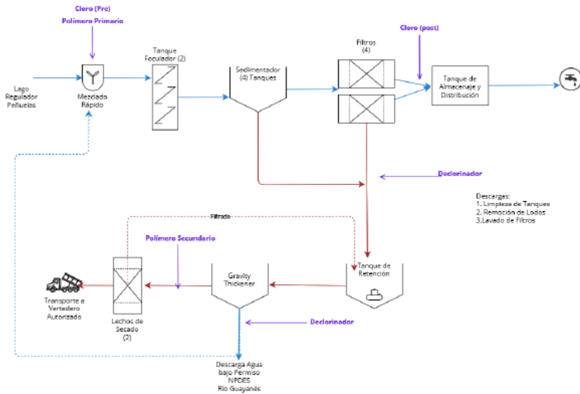
Figura 1: Esquemático Planta de Filtración y Sistema de Manejo de Lodo PF Peñuelas
