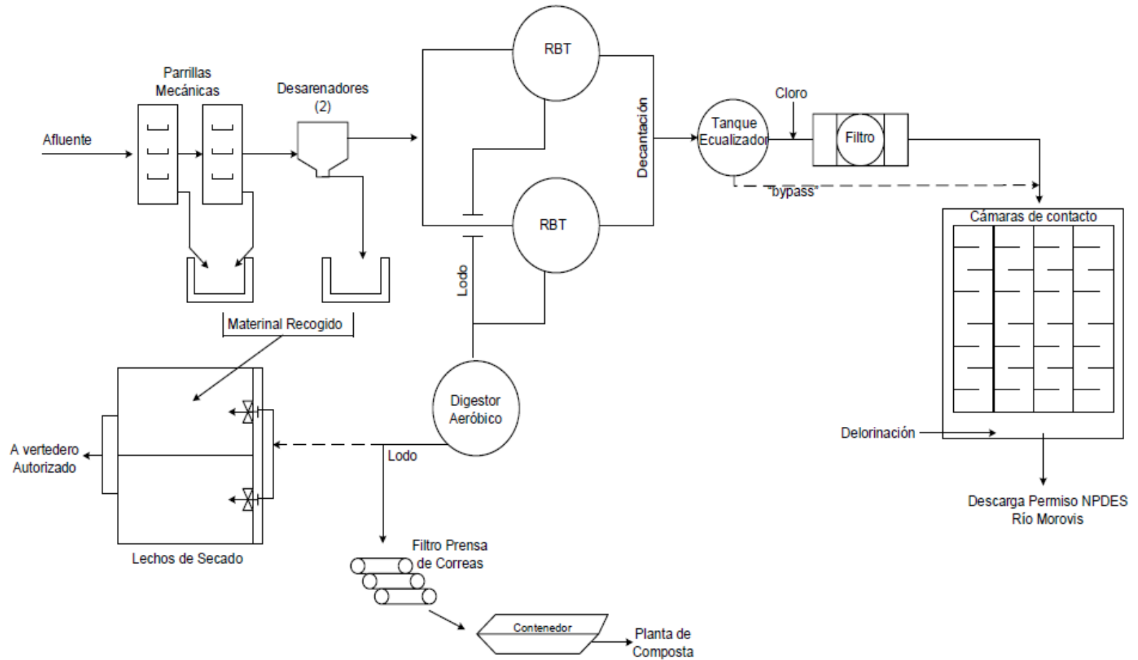
Figura 1: Esquemático Planta De Alcantarillado Sanitario de Morovis
