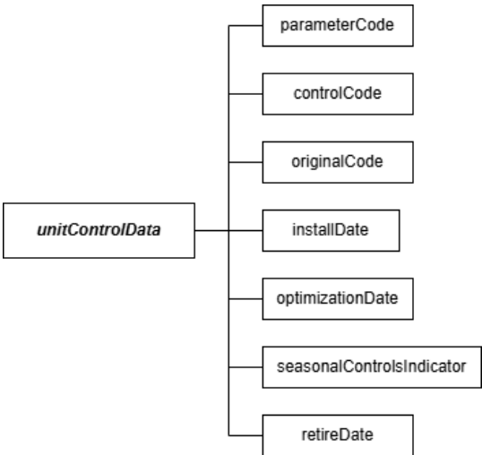
Figure 8: unitControlData JSON Elements
