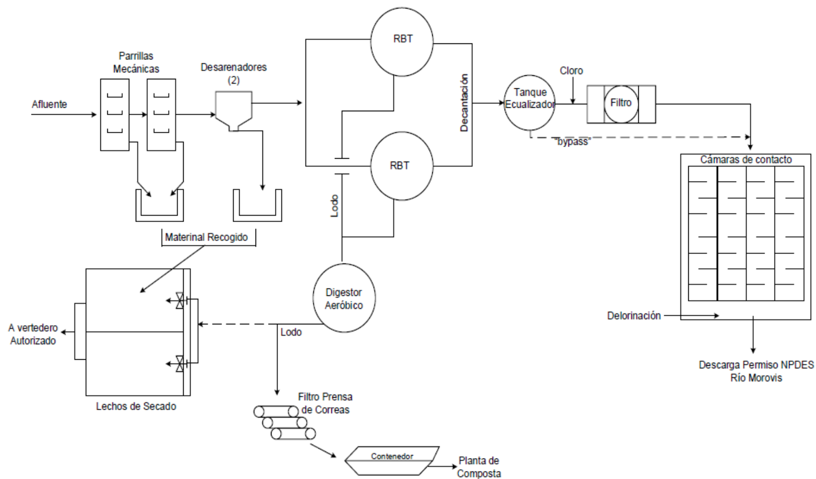
Figura 1: Esquemático Planta De Alcantarillado Sanitario de Morovis
